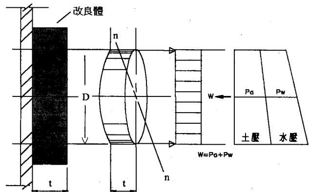
圖 5 改良長度計算方式示意圖(砂土或互層)
