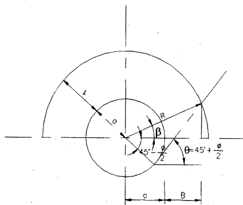
圖 9 側邊改良厚度計算方法示意圖
